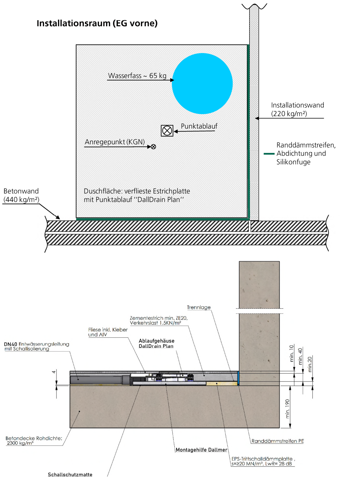
Bild oben: Lage des Prüfaufbaus im Installationsraum (EG vorne).
